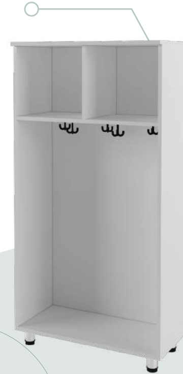
FR 49 Fores Açık Bölümlü Vestiyer Dolabı / Gardrobe with Compartment 80x40x156 h
